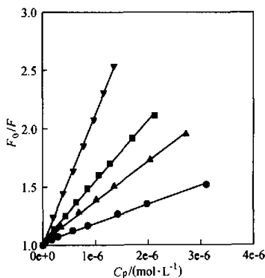
图 1 不同浓度的卟啉对 EB-DNA 荧光猝灭 ( F_0/F vs C_p )
