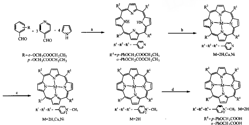
图式 1 合成路线及化合物
