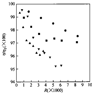
图 2 DNA 相对粘度 \eta/\eta_0 随 R 值的变化
