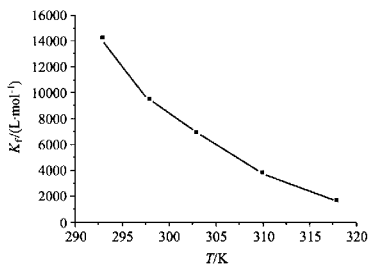
图 3 Tan II A-HPCD 包合物的形成常数 K_f 随温度的变化 Figure 3 Effect of temperature on the equalization constants K_f of complexes of Tan II A-HPCD
